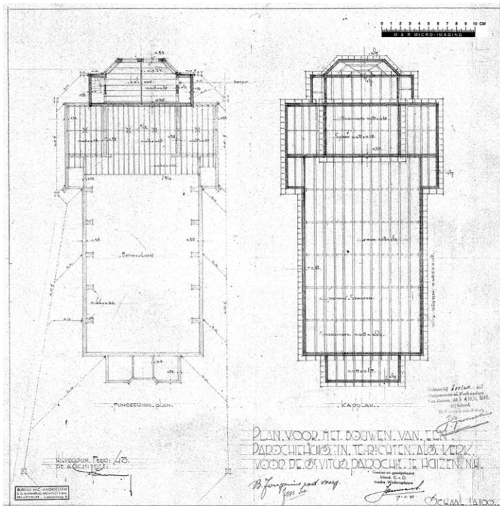
Ontwerptekeningen uit 1948 door S.G. Barenbrug (Gemeente Huizen, bouwdoossier)
