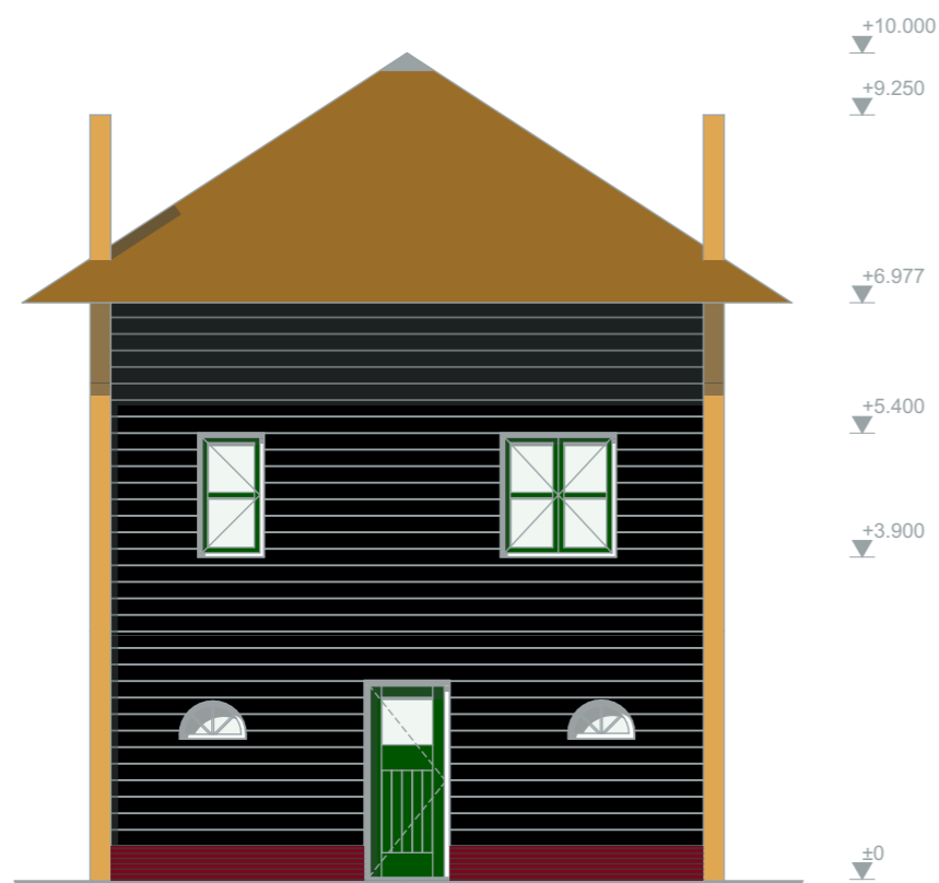
Voorgevel
