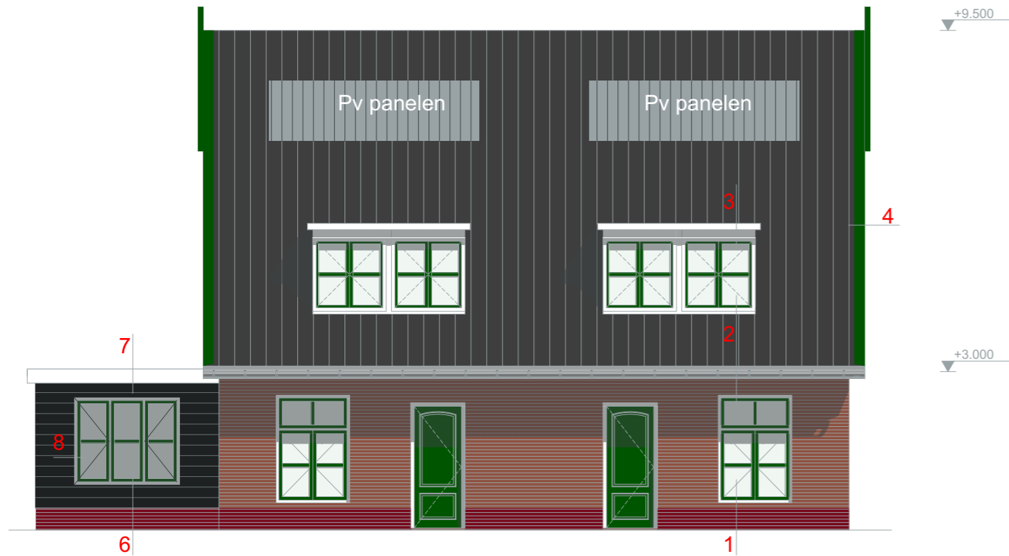
Voorgevel
