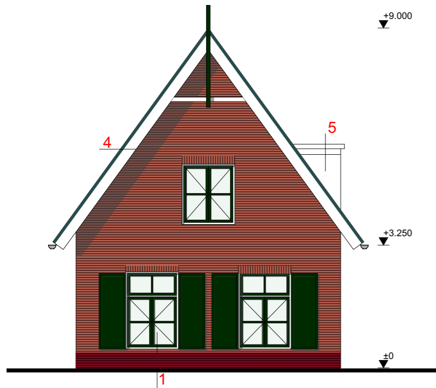
Voorgevel
