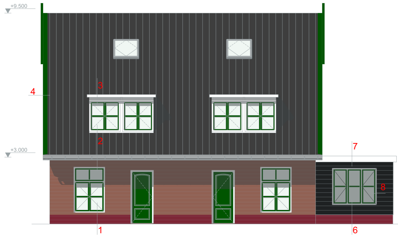
Voorgevel
