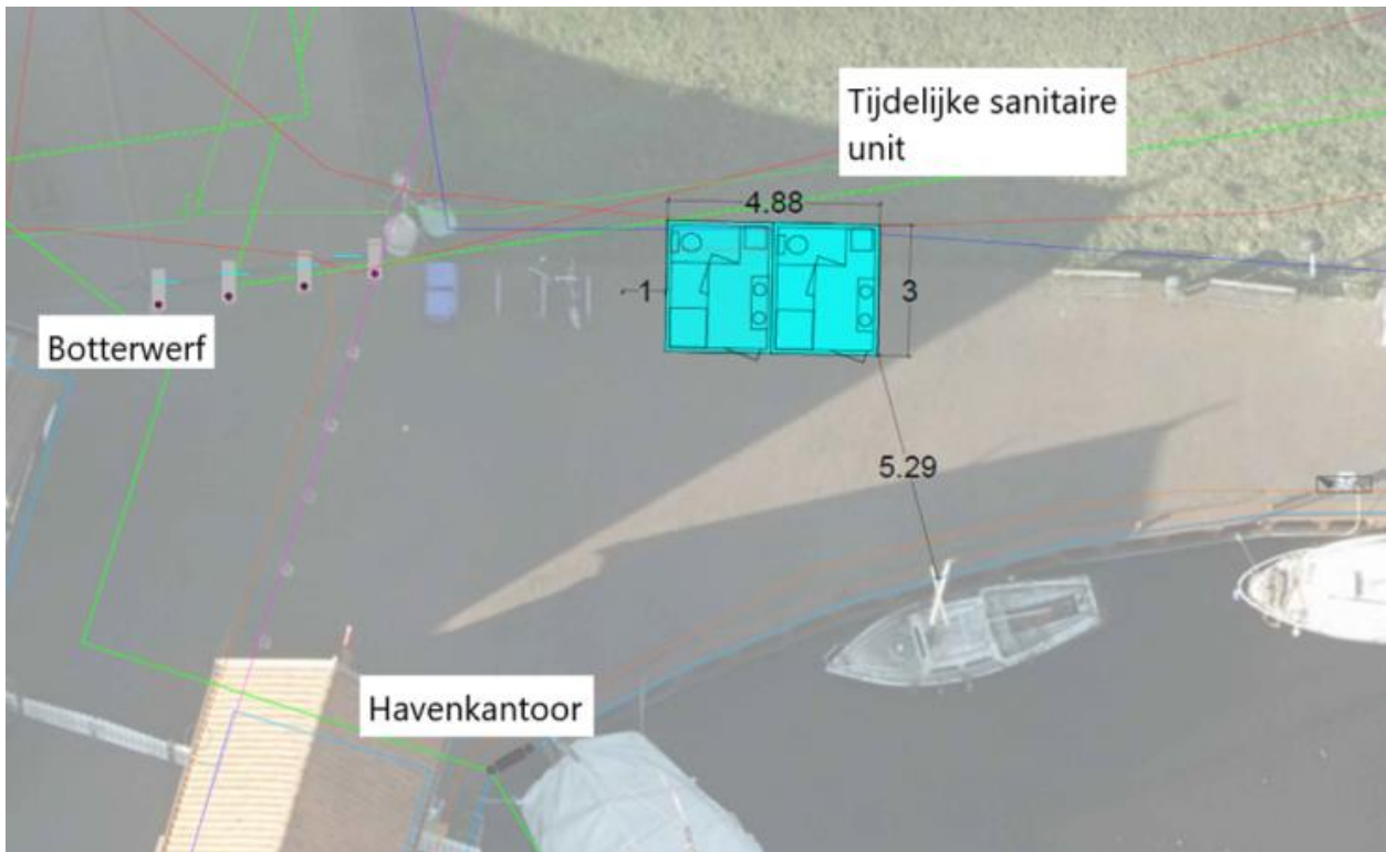
Figuur 1. Locatietekening
